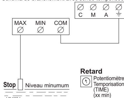
Schéma de branchement avec sonde temporisée
