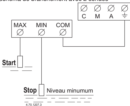
Schéma de branchement avec 2 sondes
