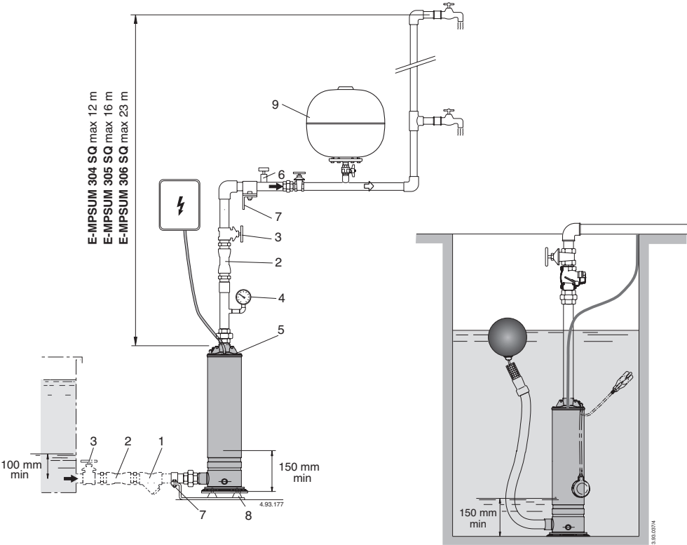
Fig. 4 Funzionamento sotto battente Positive suction head operation Fonctionnement en charge
