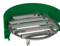
Réhausse hauteur 300 mm Barreaux anti-chute BACCD 300
