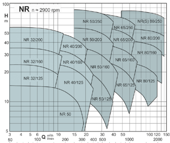
n ≈ 2900 1/min
