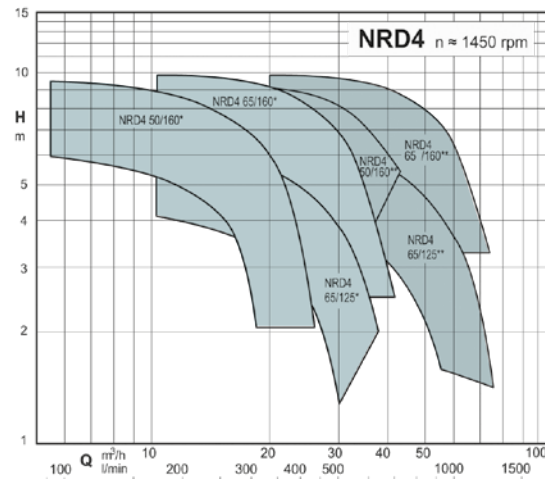
n ≈ 1450 1/min
