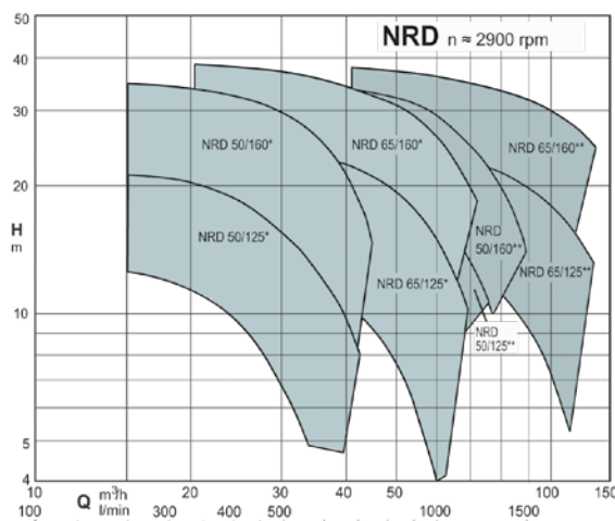
n ≈ 2900 1/min
