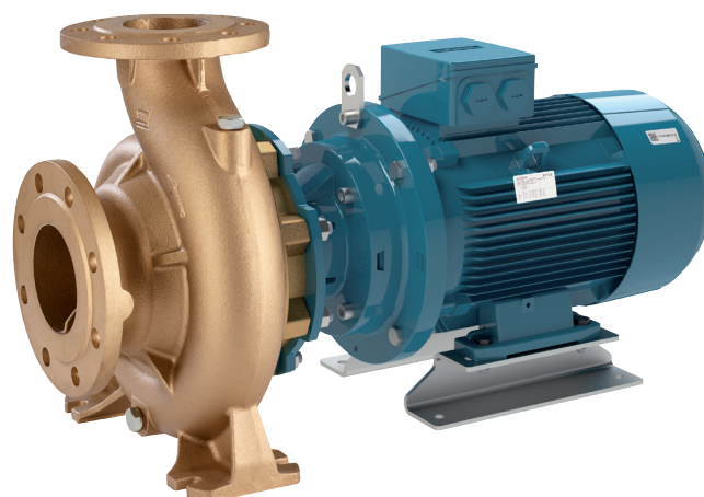
NMS, NMS4 (Ausführung Steckwellenkonstruktion in Grauguss) BNS, BNS4 (Ausführung Steckwellenkonstruktion in Bronze)
