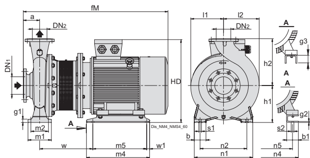
Flansche nach EN 1092-2
