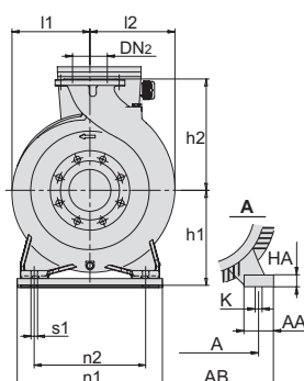
Flansche nach EN 1092-2
