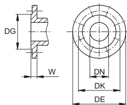
Flansche nach EN 1092-2
