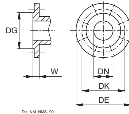
Flansche nach EN 1092-2
