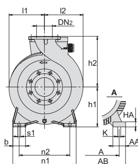
Flansche nach EN 1092-2
