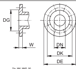
Flansche nach EN 1092-2
