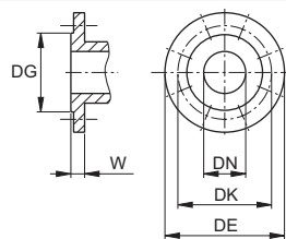
Flansche nach EN 1092-2
