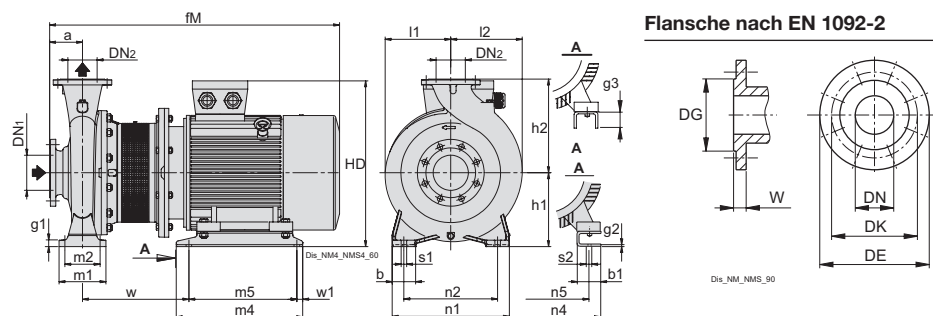
Flansche nach EN 1092-2
