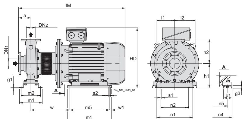
Flansche nach EN 1092-2
