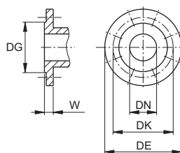
Flansche nach EN 1092-2
