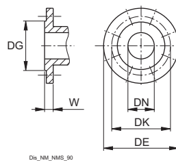
Flansche nach EN 1092-2
