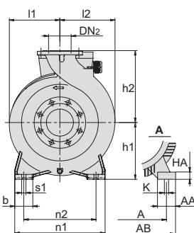
Flansche nach EN 1092-2
