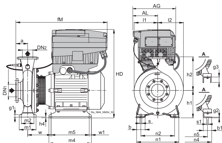
Flanges EN 1092-2
