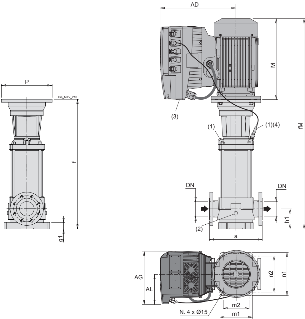
Bridas EN 1092-2
