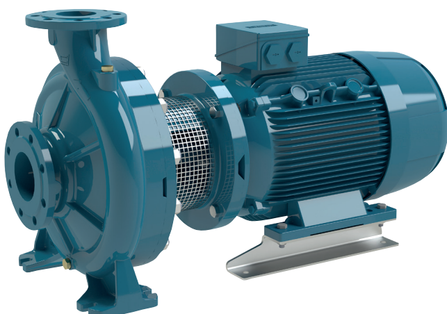
NMS, NMS4 (versión Stub-shaft de hierro)
