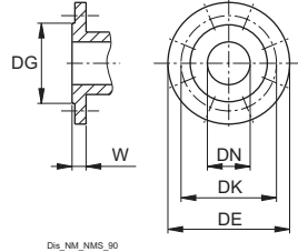
Bridas EN 1092-2
