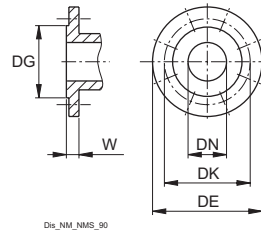
Bridas EN 1092-2
