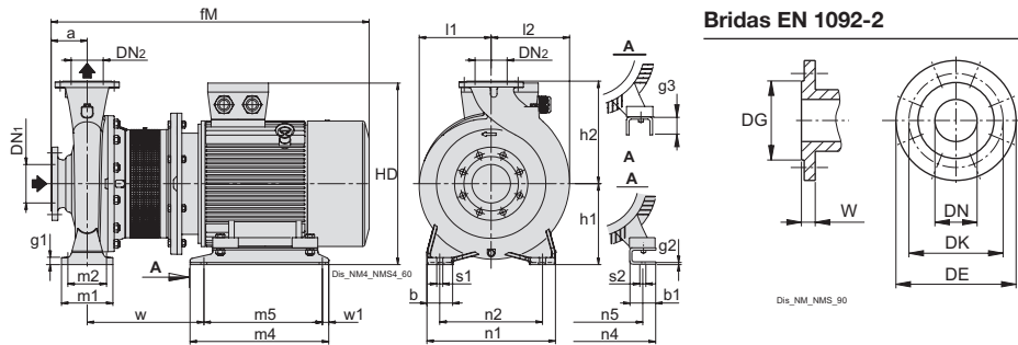
Bridas EN 1092-2
