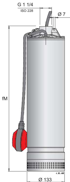
MPSM ... CG Pompe con galleggianti (a richiesta).
