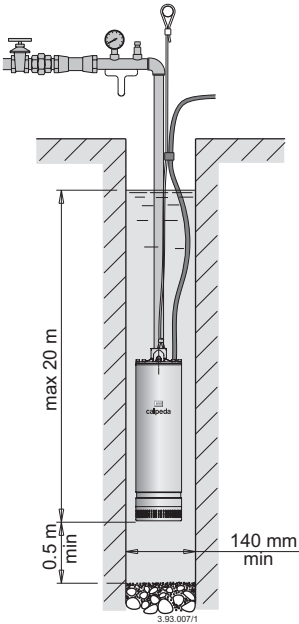
Pompa sospesa
