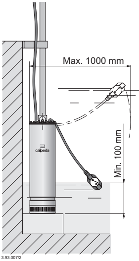
Pompa appoggiata
