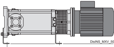
Installazione orizzontale.
