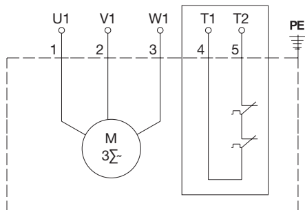
Conexión Tres fases 230V / 400V
