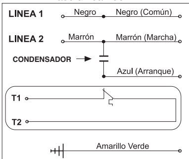
Conexión Fase única 230V
