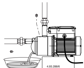
Fig. 5 Scarico Draining Entleerung Vidange Vaciado Avtappning Aftappen Αποστράγγισι Слив 排空
