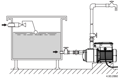
Fig. 1 Funzionamento sotto battente Positive sition head operation Zulaufbetrieb Fonctionnement en charge Funcionamiento bajo carga Tillrinning sugsidan Toeloopsituatie Θέση λειτουργίας με θετική αναρρόφηση Работа под гидравлическим напором 正吸上水头的操作
