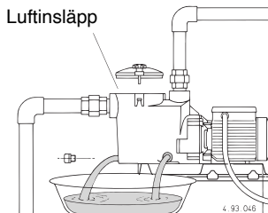
Fig. 4 Dränering
