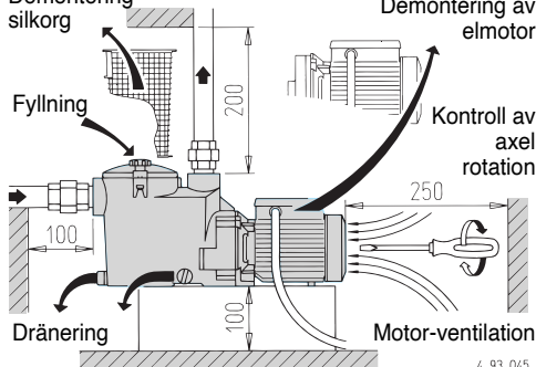
Fig. 1 Minimum utrymme för service (mm)
