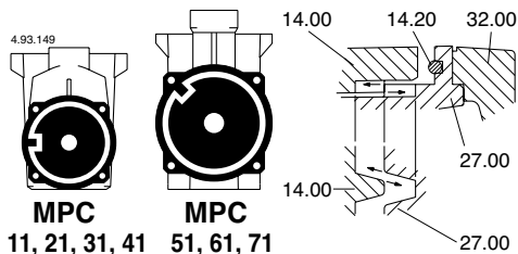
Abb. 6 MontagenunterZusammenbauPumpengehäuse (14.00) - Diffusordeckel (27.00)
