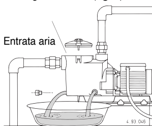
Fig. 4 Scarico
