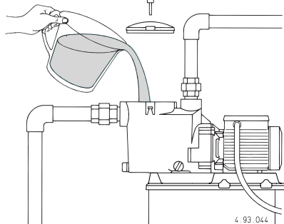
图2 灌泵
