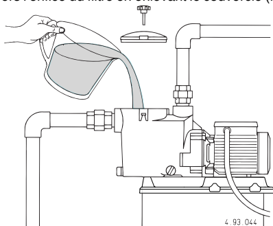
Fig. 2 Remplissage
