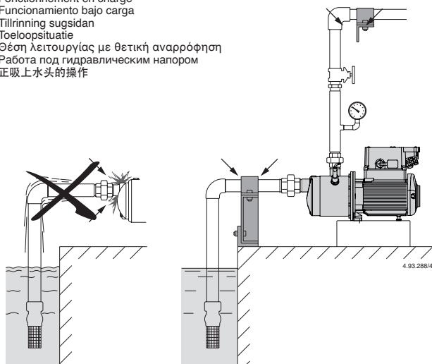
Fig. 3 Sostegni ed ancoraggi delle tubazioni Supports and clamps for pipelines Stützen und Verankerungen der Rohrleitungen Soutien et ancrage des tuyaux Sostén y anclaje de la instalación Konsoll samt klämmor för rör Steunen voor leidingen Υποστήριξη και σφίξιμο σωληνώσεων Опоры и крепления труб 管路的支撑及夹具
