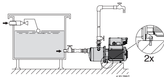
Fig. 1 Funzionamento sotto battente Positive suction head operation Zulaufbetrieb Fonctionnement en charge Funcionamiento bajo carga Tilrinning sugsidan Toeloopsituatie Θέση λειτουργίας με θετική αναρρόφηση Работа под гидравлическим напором 正吸上水头的操作
