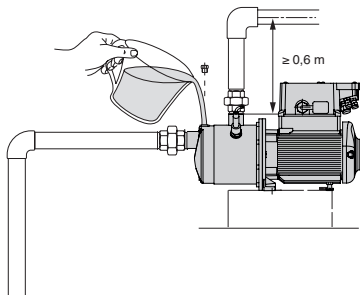
Fig. 4 Riempimento Filling Auffüllung Remplissage Llenado Fyllning Vullen Γέμιση Наполнение 灌泵
