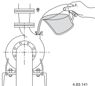
Rys. 3 Napełnienie.
