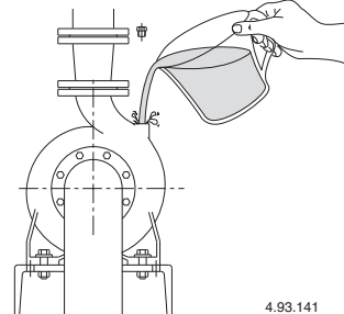
Рис. 3 Заполнение жидкостью
