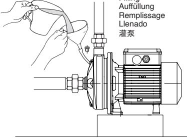
Fig. 4 Scarico Draining Entleerung Vidange Vaciado 排空
